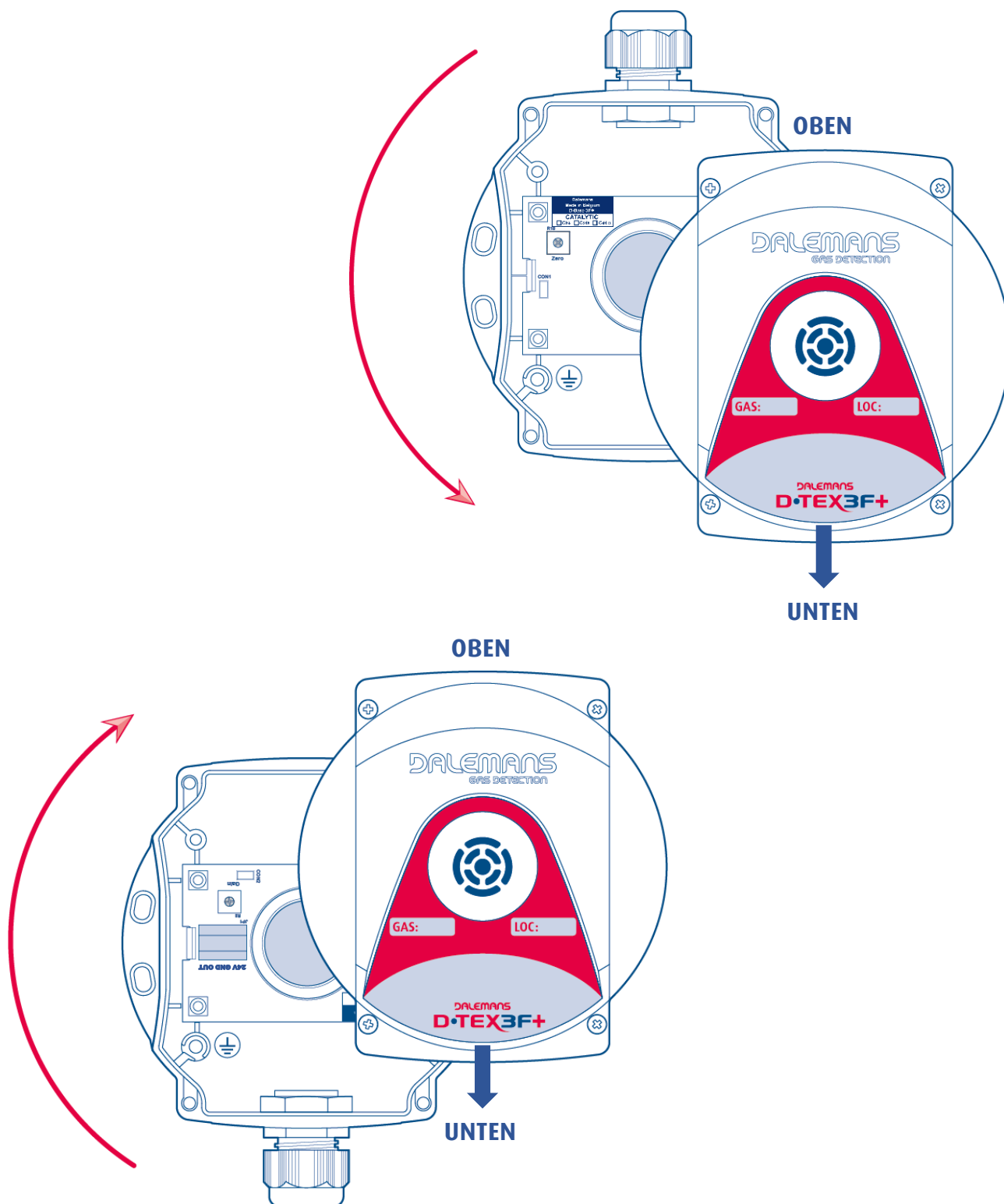
Abbildung 4: vertikale Montage des D•TEX3F+
